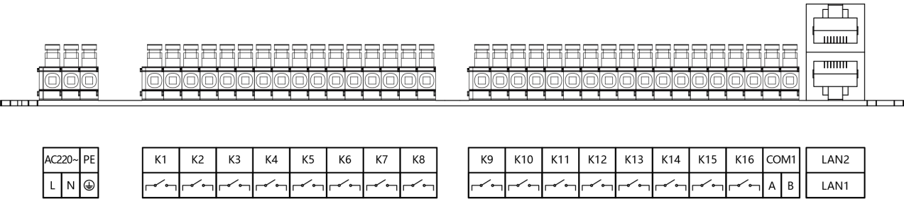
多功能控制单元接线指示图 Multifunctional control unit wiring instruction diagram
