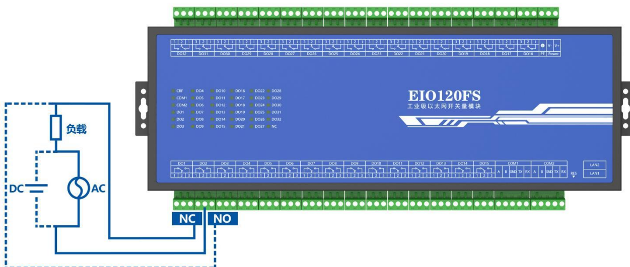
常开/常闭 继电器输出接线示意图
