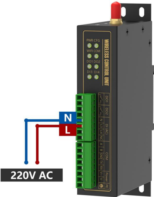
电平信号输入接线示意图
