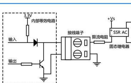
接固态继电器示意图
