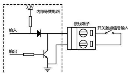
开关触点信号输入接线示意图
