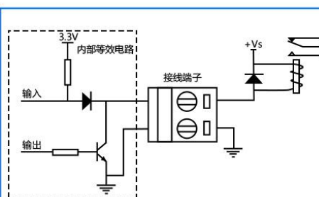
接电磁继电器示意图
