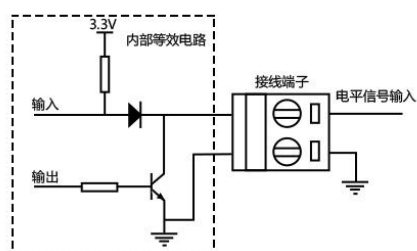
电平信号输入接线示意图
