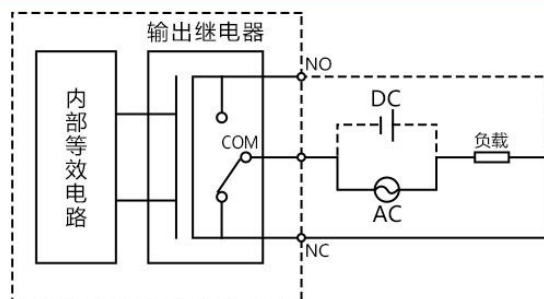
常开/常闭 继电器输出接线示意图
